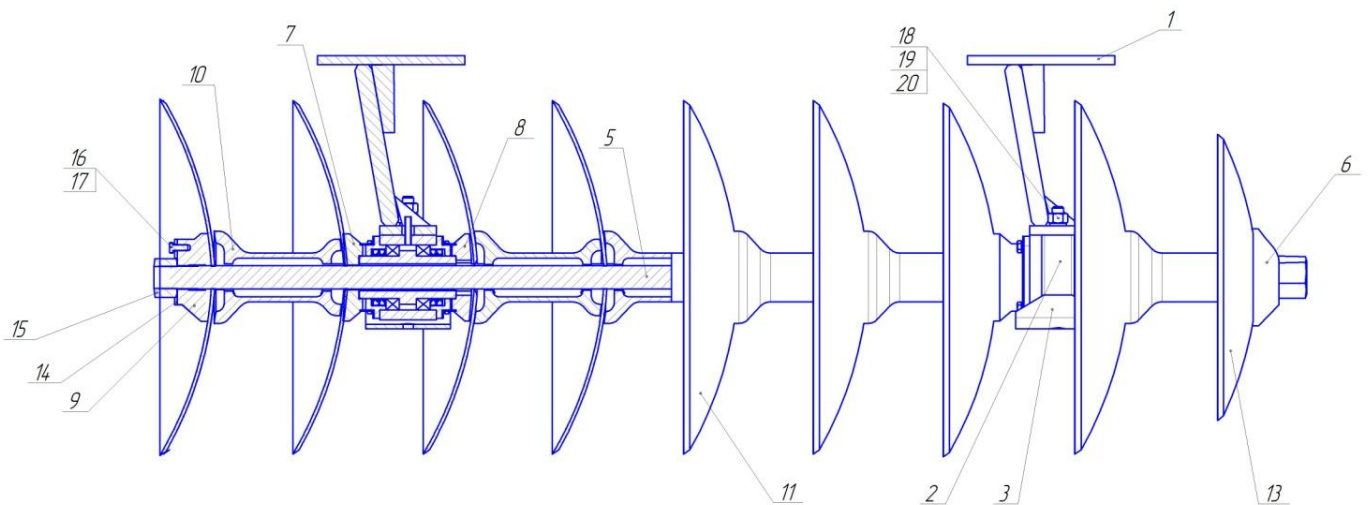
БДС.10.00.000-03.СБ 9-и дисковая батарея.
